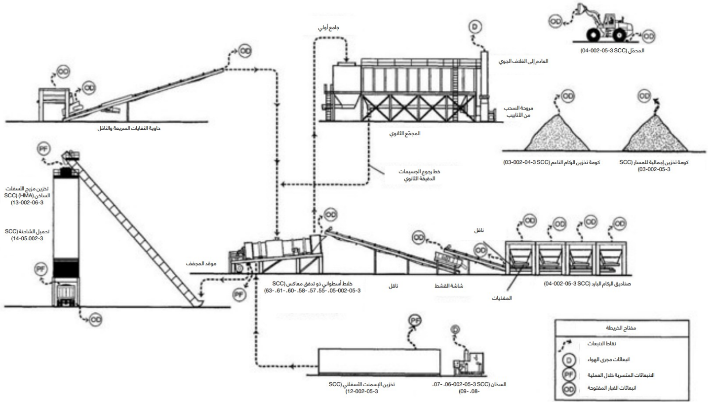
الصورة 1: مثال على عملية مصنع مزيج الأسفلت الساخن
